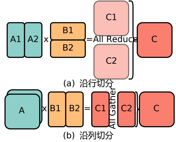
Fig. 3 张量并行
