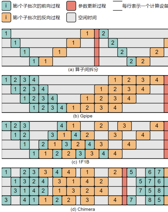
Fig. 5 流水线并行
