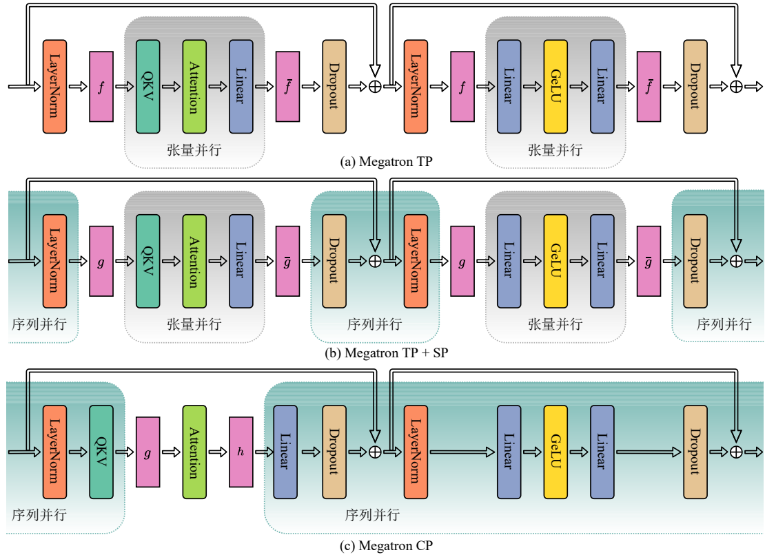
Fig. 4 张量并行与序列并行示意图
